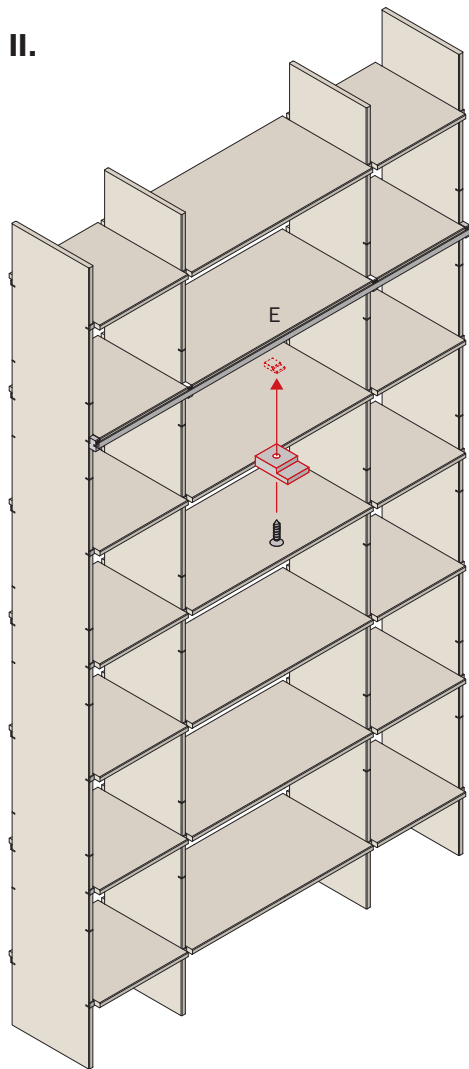
Beispiel 2 / example 2 FNP Regal mit breiten Tablaren FNP shelf with wide shelf boards
